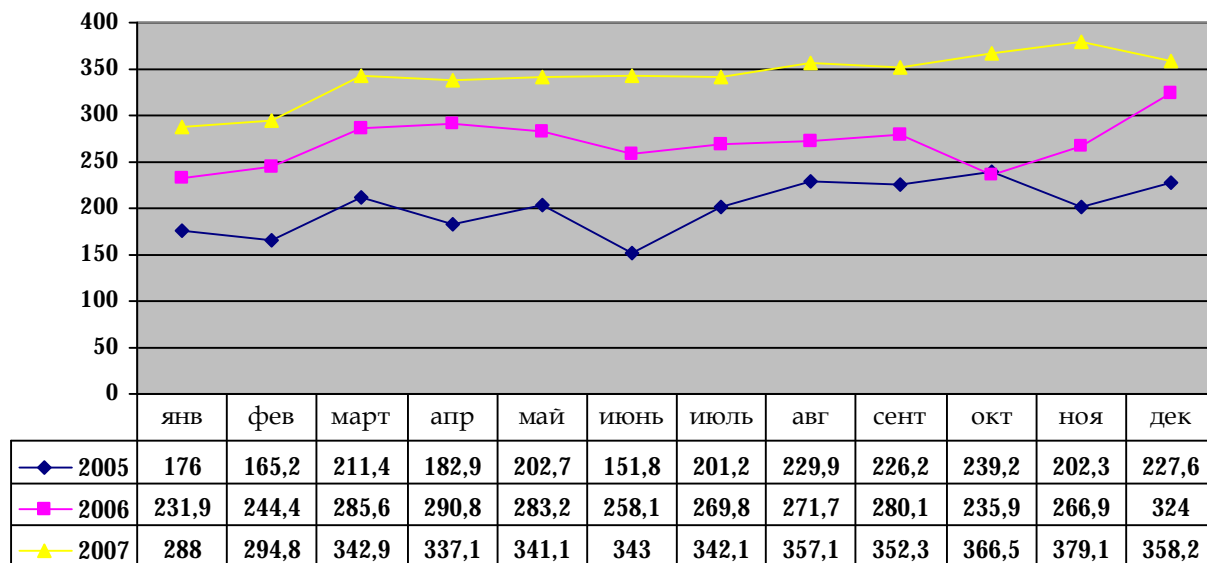
Производство электротехнической стали 2005-2007 гг по месяцам, тыс т
