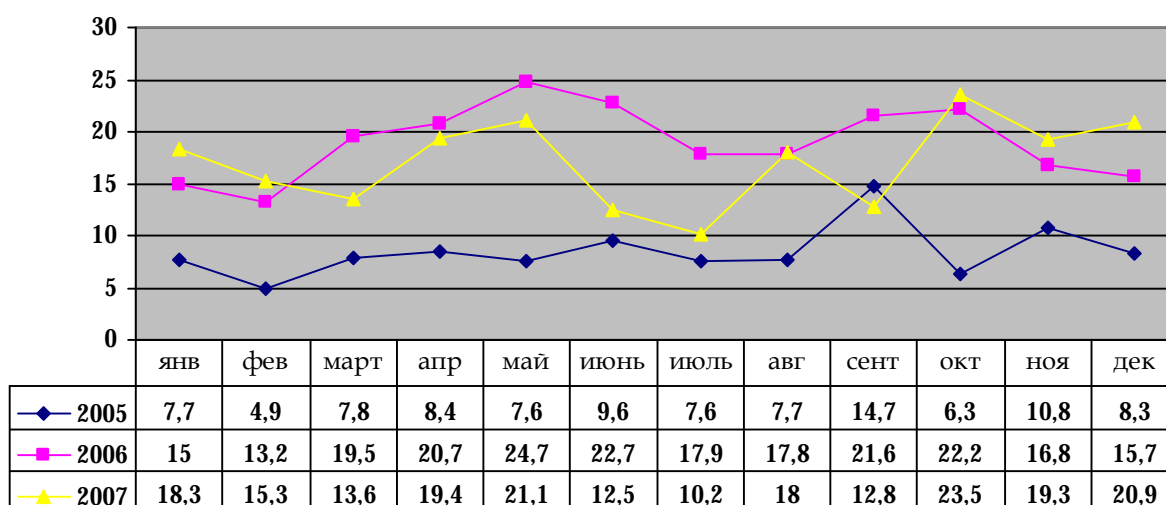
Экспорт ЭТС с 2005 по 2007 гг по месяцам, тыс т
